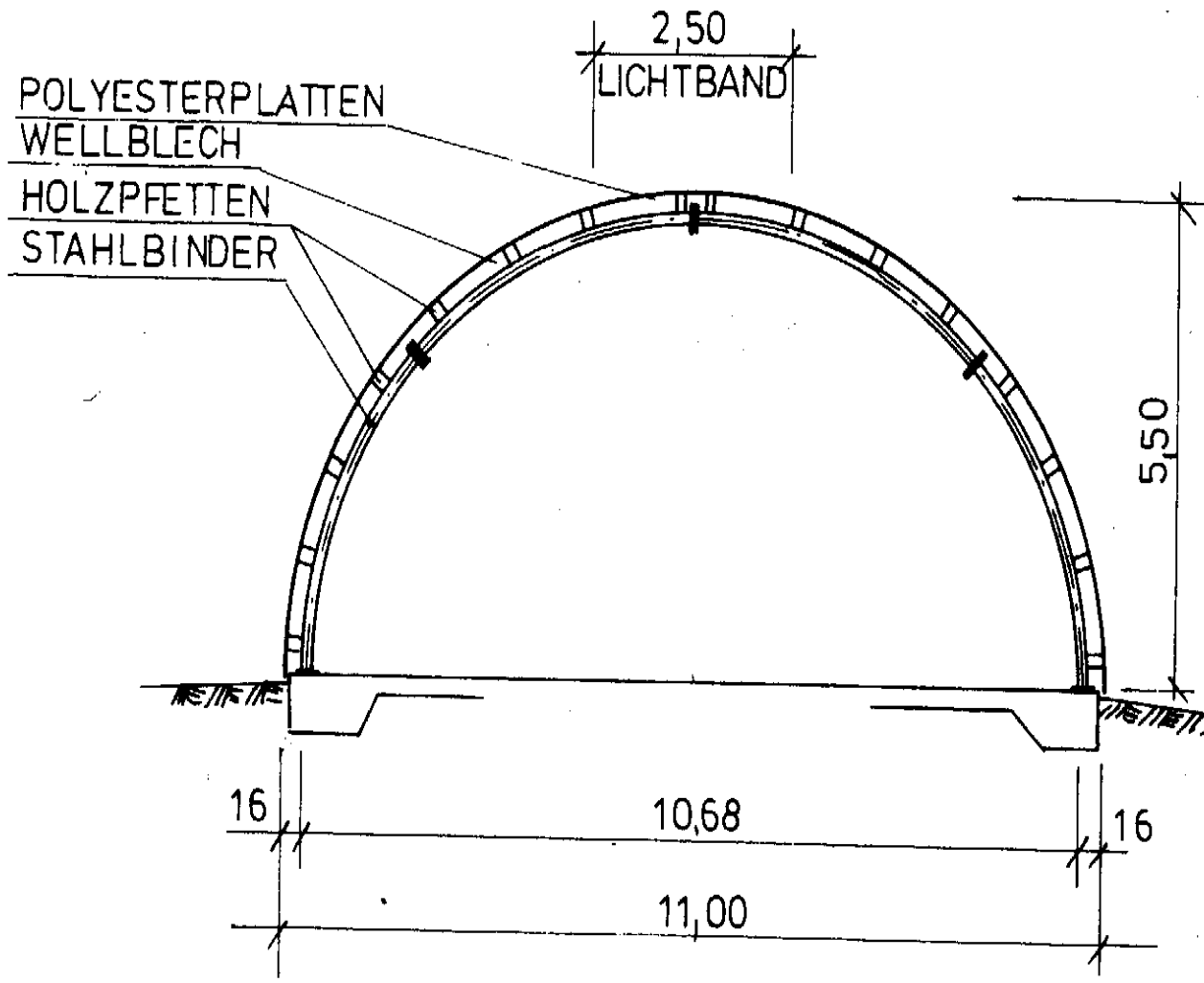
QUERSCHNITT
