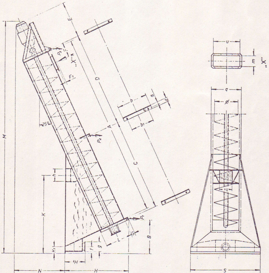
Sand-, Wasch- u. Entwässerungsschnecken 400 - 700 Schneckendurchmesser
