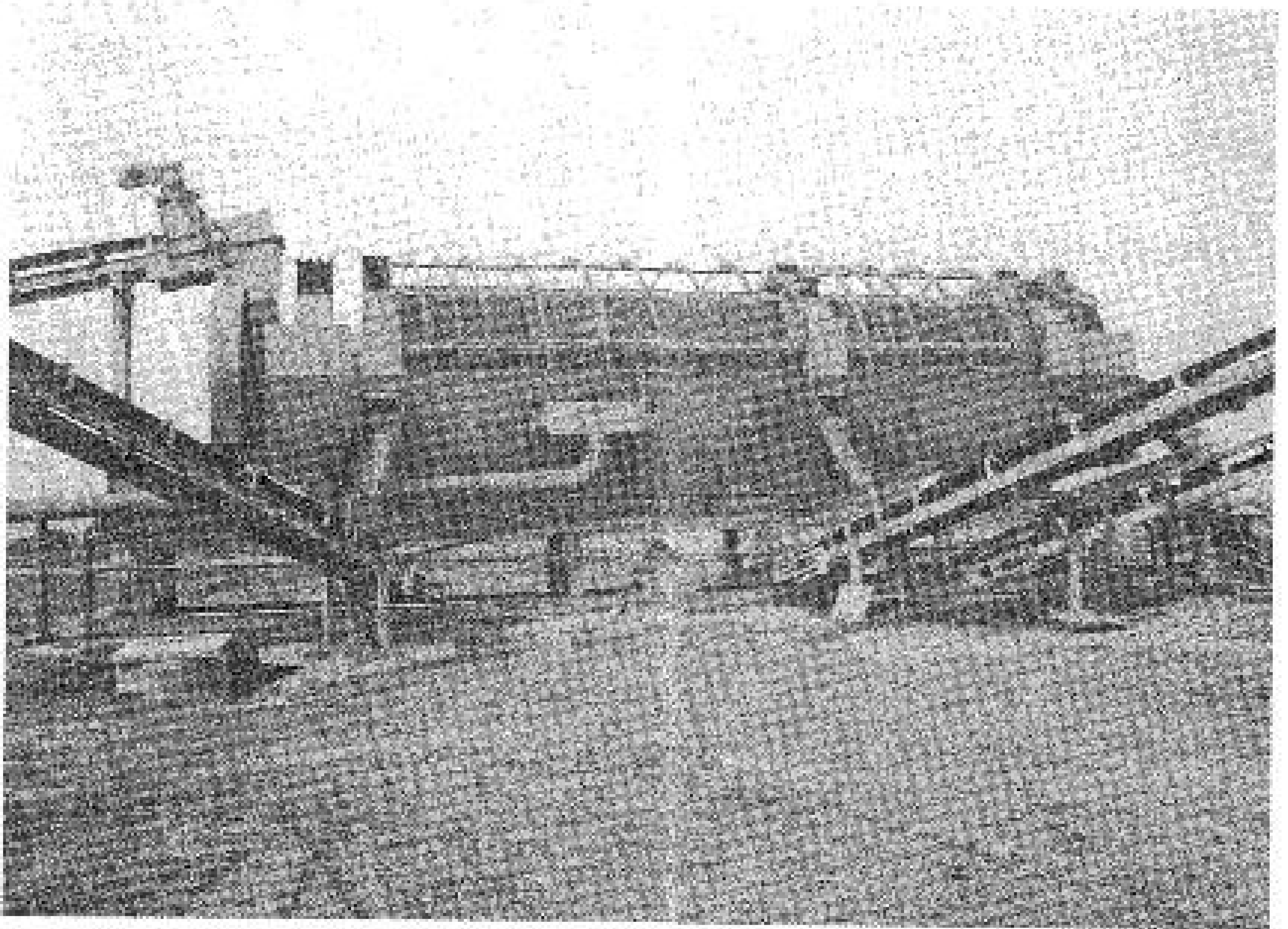
Abb. 53: Trogwaschmaschine
