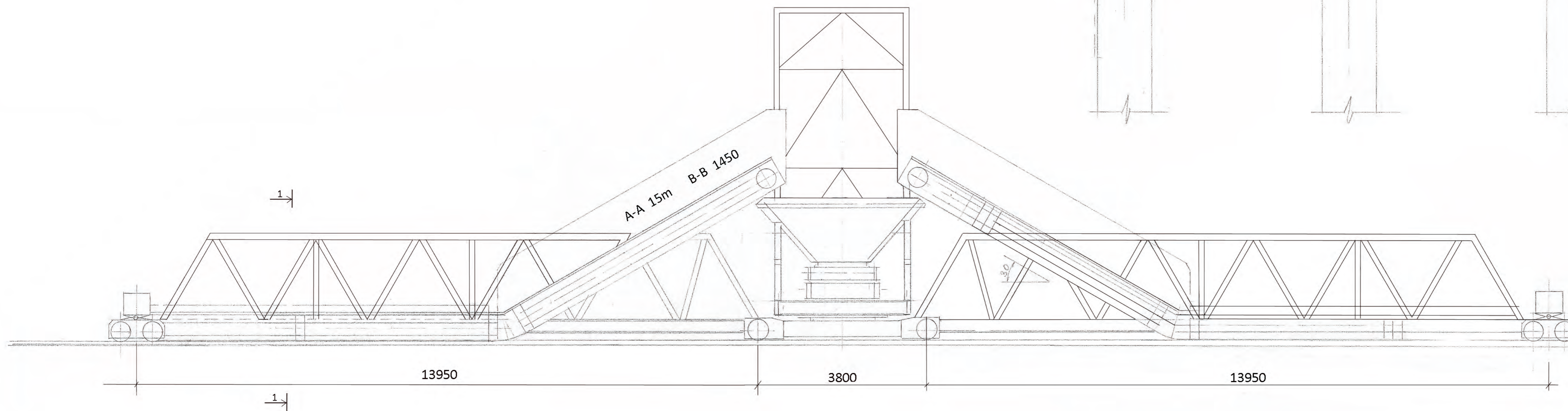
ANSICHT B-B
