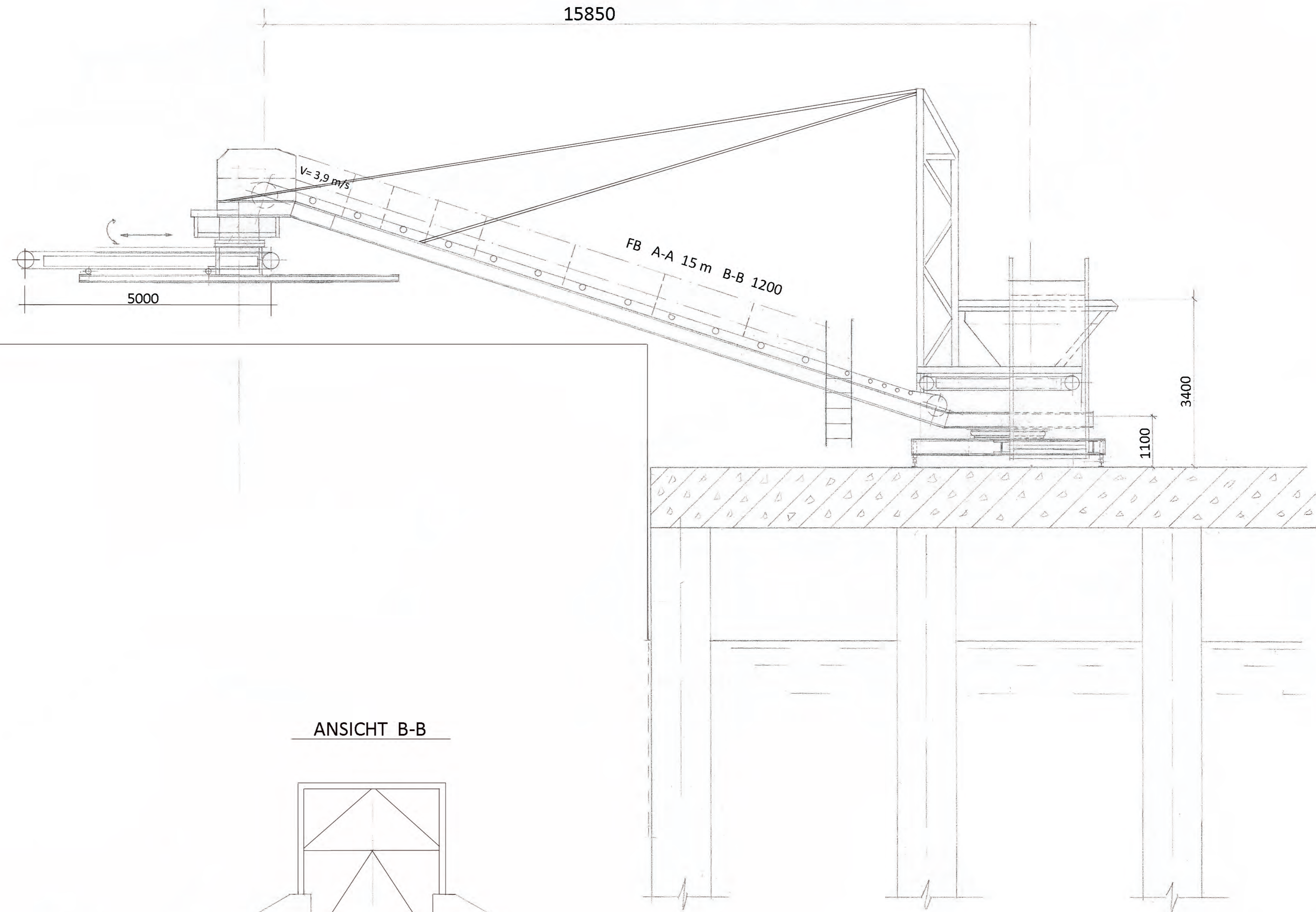
ANSICHT A-A
